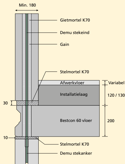
DRAGENDE GEVELWAND VERDIEPING
