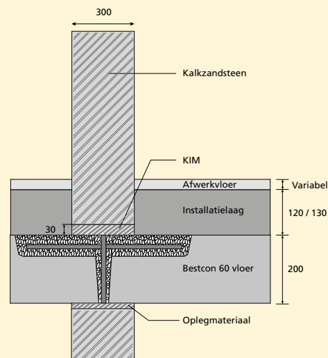
DRAGENDE BINNENWAND, VERDIEPING WONINGSCHIEDEND
