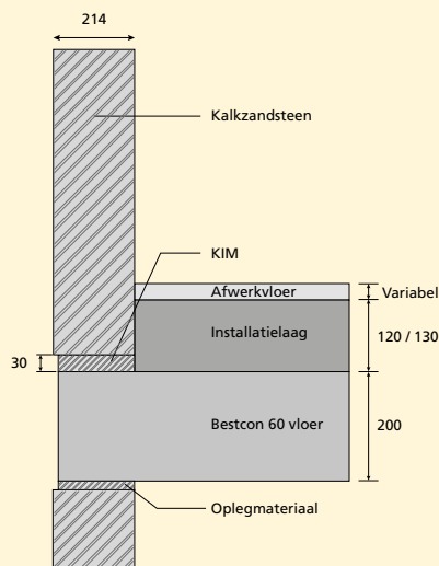
DRAGENDE GEVELWAND VERDIEPING
