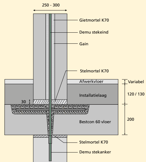
DRAGENDE BINNENWAND, VERDIEPING WONINGSCHIEDEND
